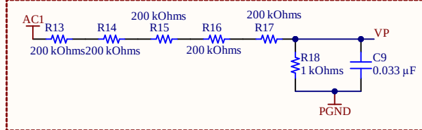
Volatge sense Resistors
